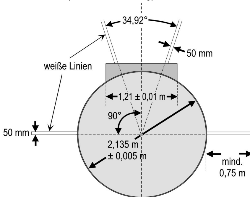
Zeichnung 18: Kugelstoßkreis
