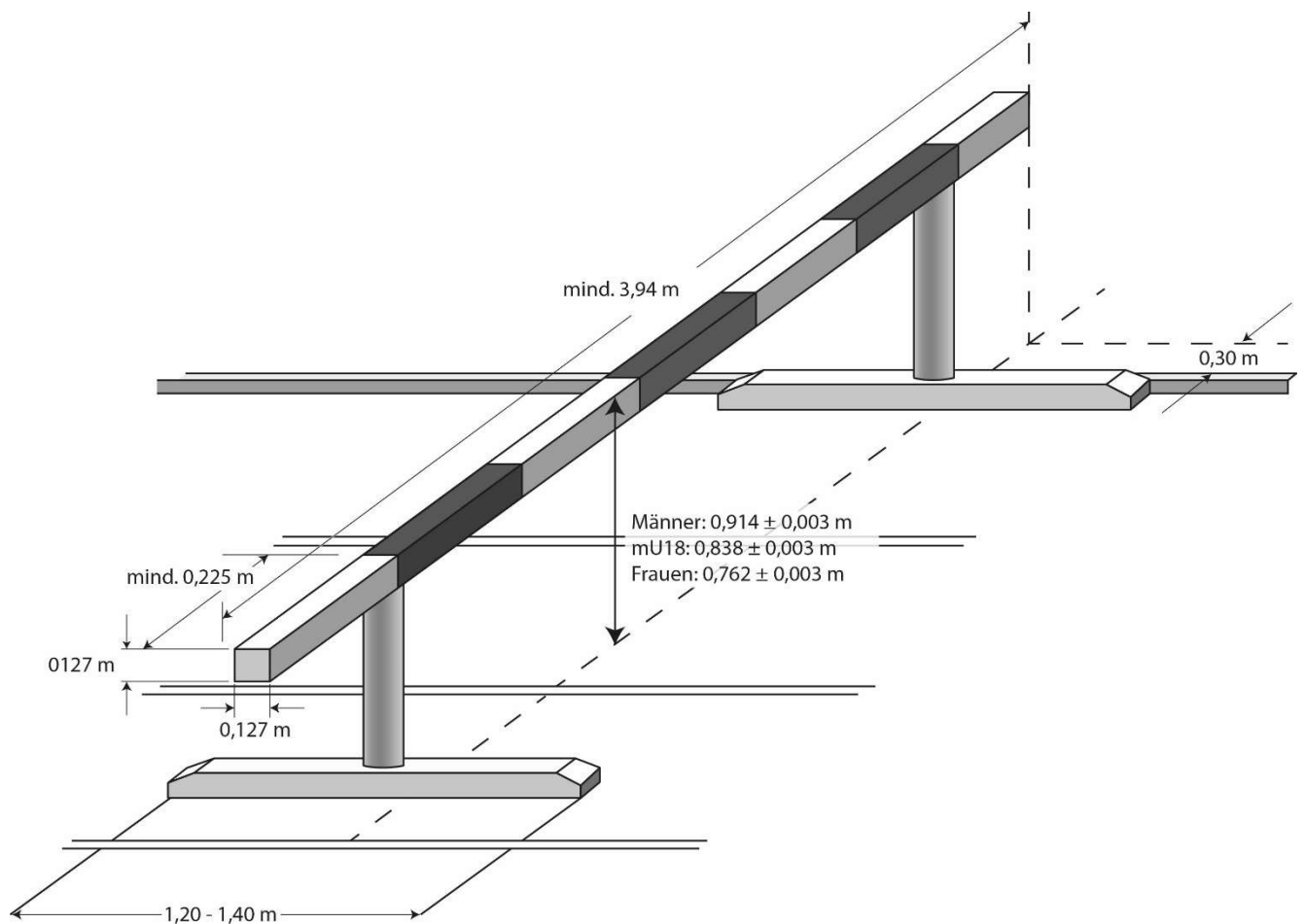
Zeichnung 6: Hindernisabmessungen
