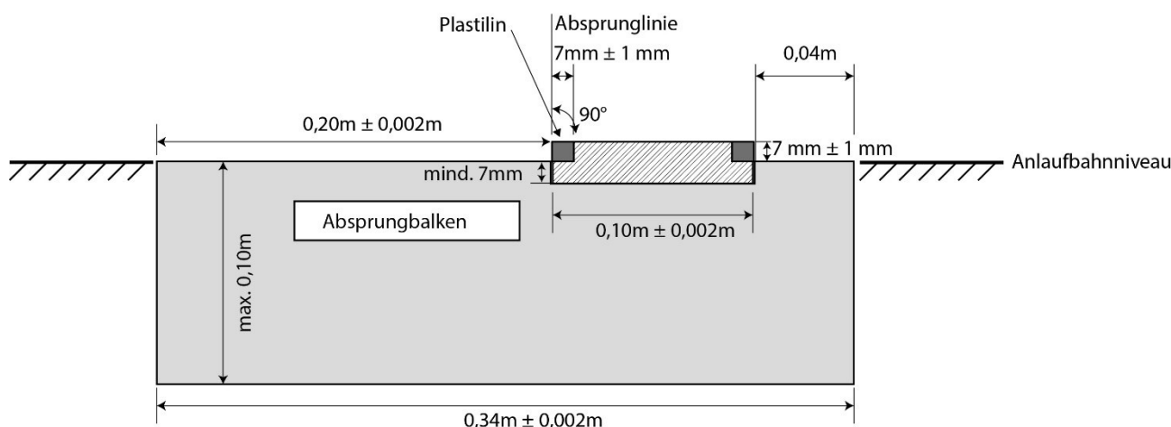
— Anlaufrichtung —> Zeichnung 14: Absprungbalken und Einlagebrett
