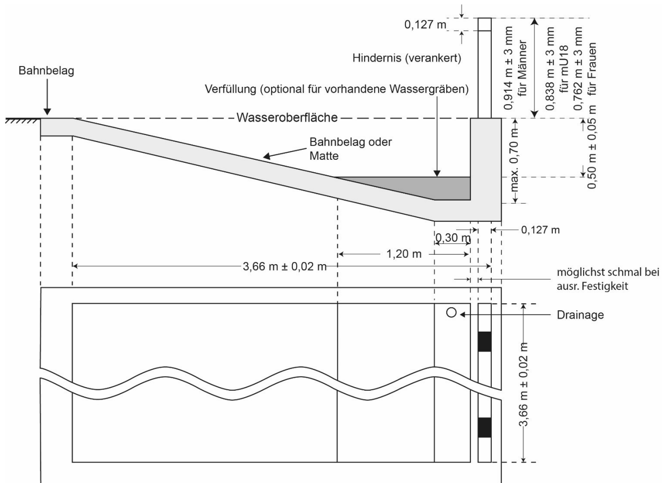
Zeichnung 7: Wassergraben
