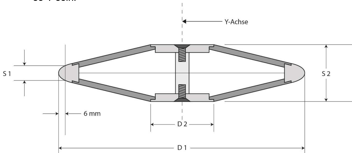
Zeichnung 27: Diskus
