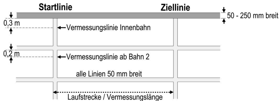
Zeichnung 1: Vermessung der Rundbahn
