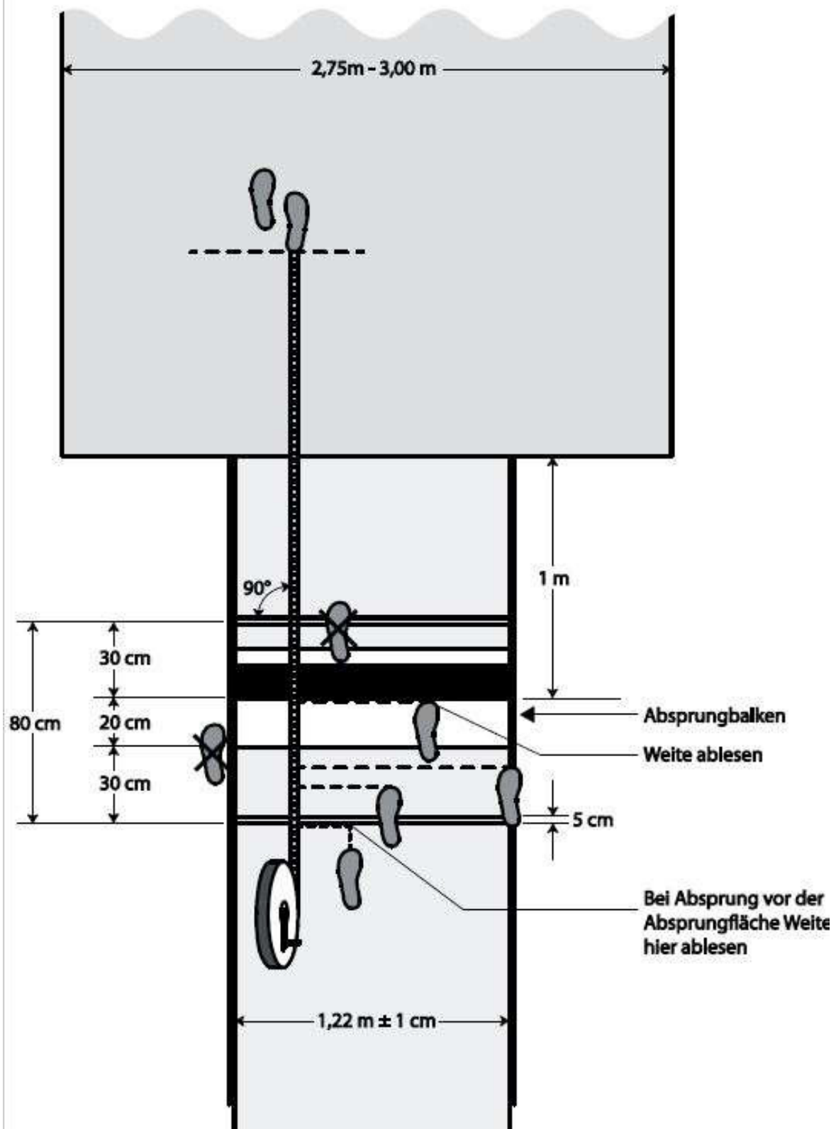
Zeichnung 17: Absprungsfläche für Weitsprung
