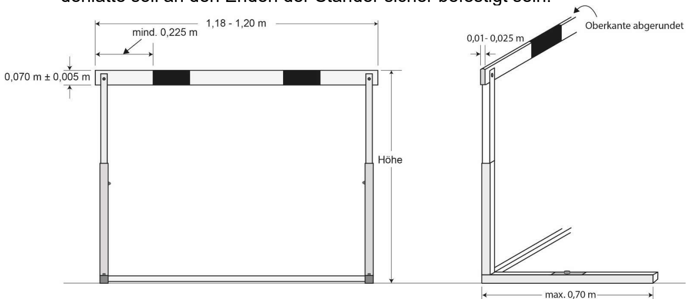
Zeichnung 4: Hürdenabmessungen
