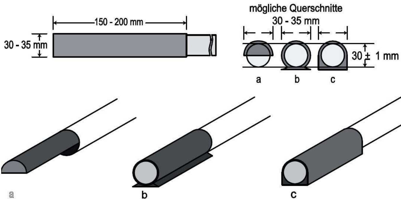
Zeichnung 8: Zulässige Endstücke der Sprunglatte
