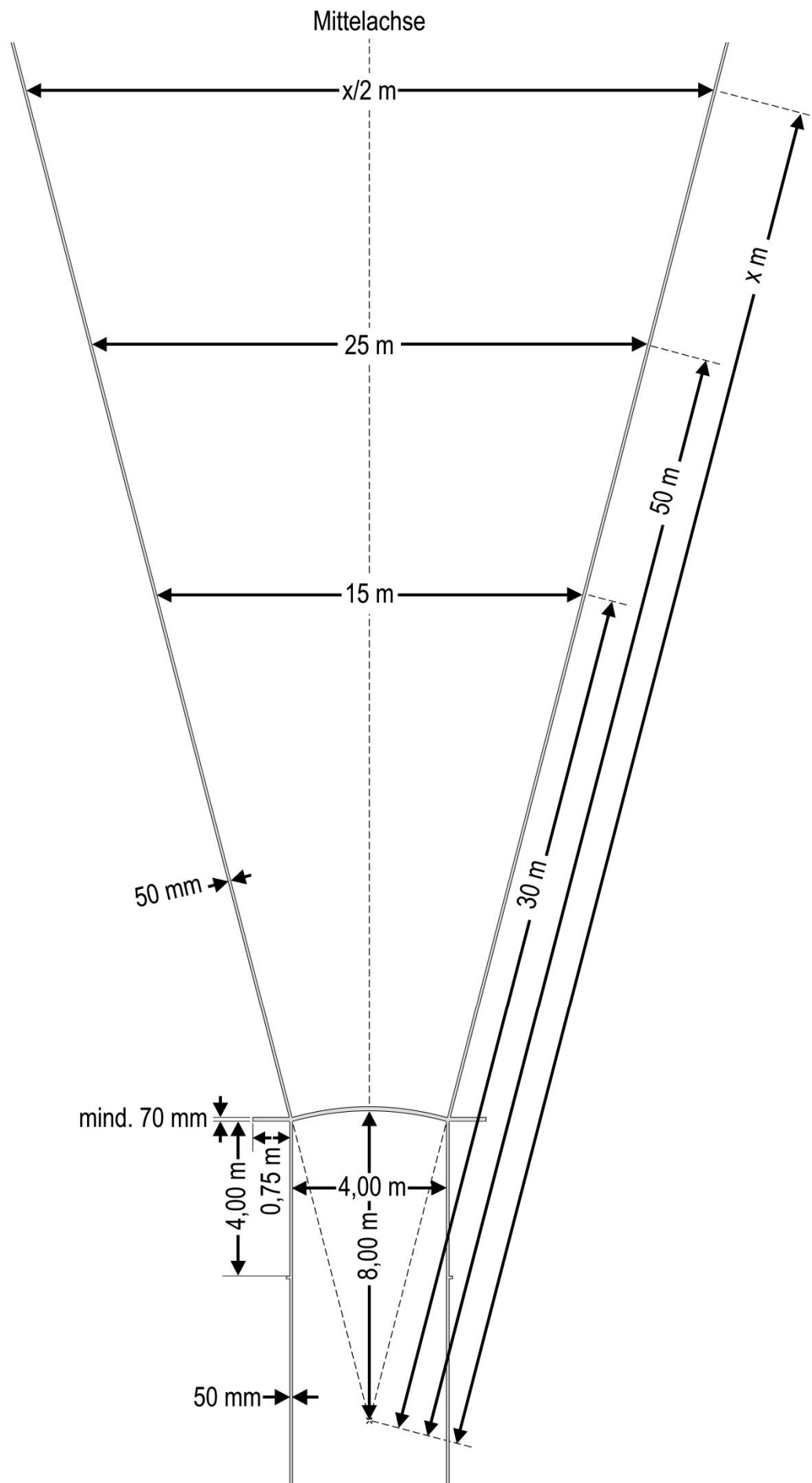
Zeichnung 24: Speerwurfsektor
