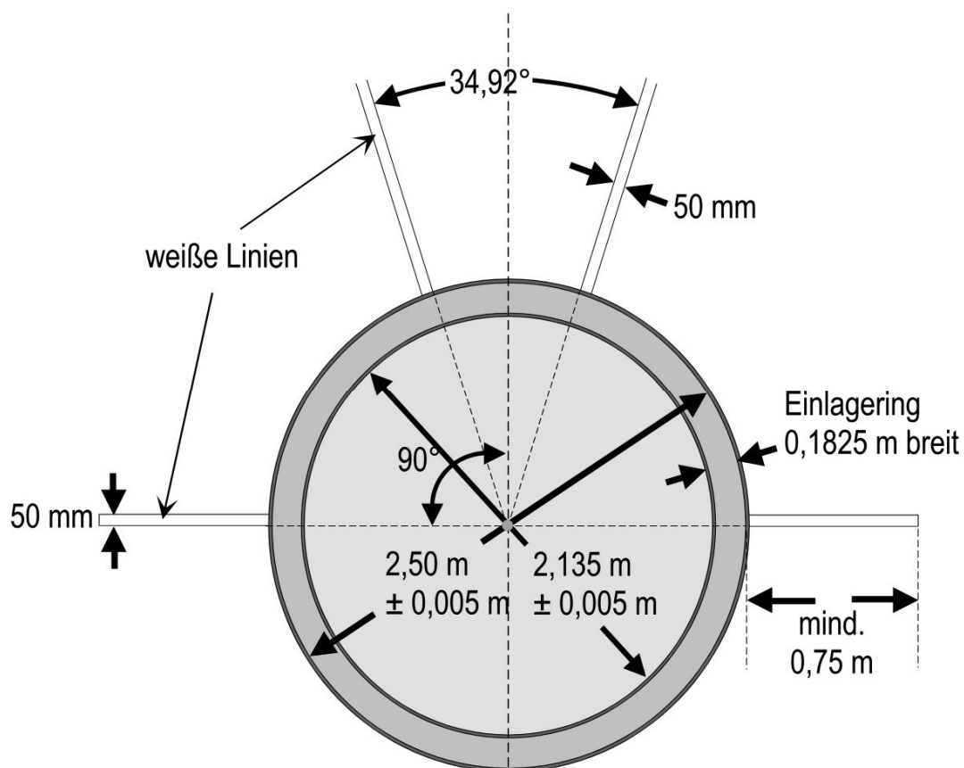
Zeichnung 21: Kombierter Diskus- und Hammerwurfkreis
